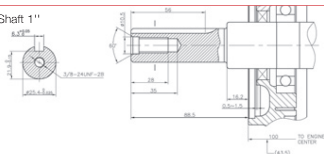
G-Shaft
